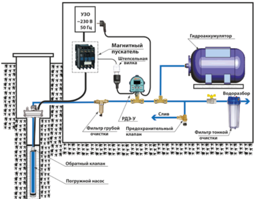
Пример 4. Подключение РДЭ-У для управления однофазным насосом мощностью P1 более 1,5 кВт, или трехфазным погружным насосом.
