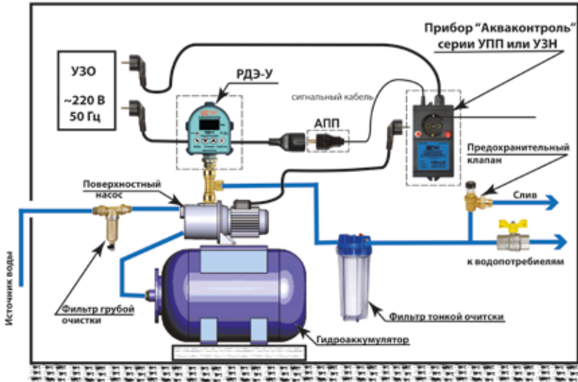
Пример 3. Подключение РДЭ-У к УПП или УЗН “Extra Акваконтроль” через адаптер АПП.
