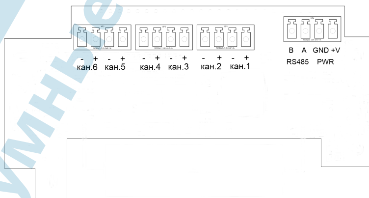
Рис. 7.2 Схема клеммников платы
