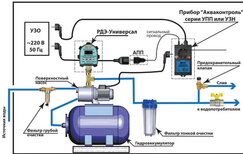
Пример 4. Подключение РДЭ-Универсал для управления однофазным насосом мощностью P1 более 1,5 кВт, или трехфазным погружным насосом.
